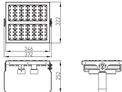
외형도
